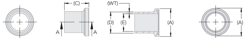
Section A-A
